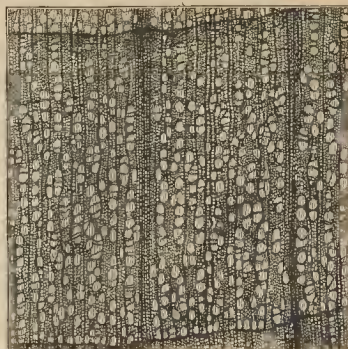
Fig. 3. - Aliso blanco ( Alnus incana , D.C.). - Sección transversal. Aumento 30 diámetros.
